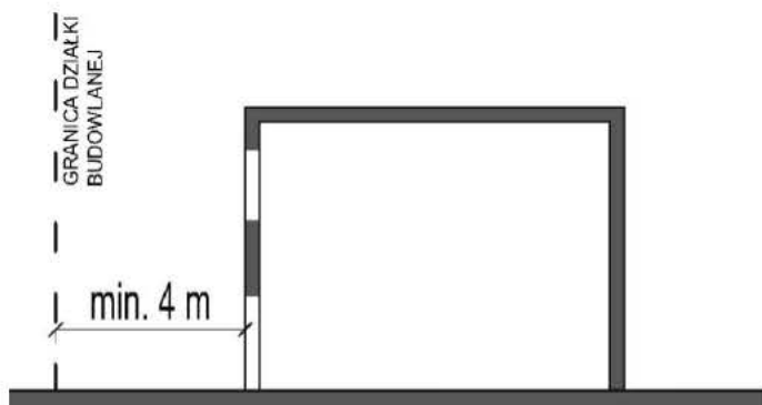
Rys. 2 Budynek zwrócony ścianą z oknami lub drzwiami w stronę granicy działki budowlanej – § 12 ust. 1 pkt 1.
